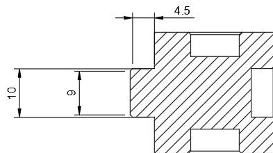
A-A (2:1)
